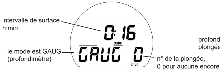
ÉCRAN PRINCIPAL DU MODE SURFACE GAUGE (pas encore de plongée ou intervalle de surface SI > 10 min)
