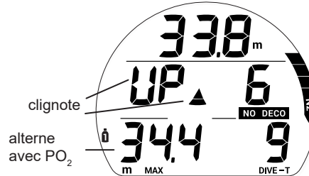
APRÈS UNE ALARME SONORE
