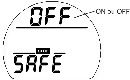
RÉGLAGE D'UN PALIER DE SÉCURITÉ SS
